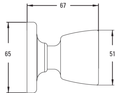
DIMENSIONES (mm)
