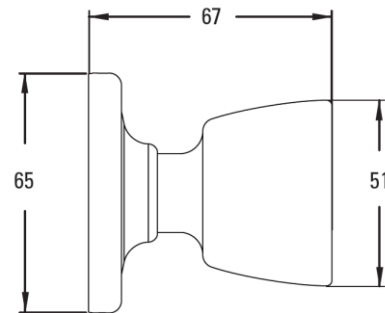
DIMENSIONES (mm)
