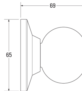
DIMENSIONES (mm)
