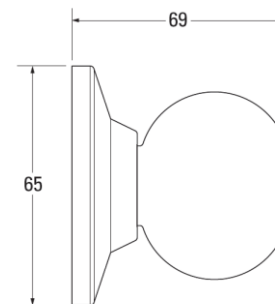
DIMENSIONES (mm)
